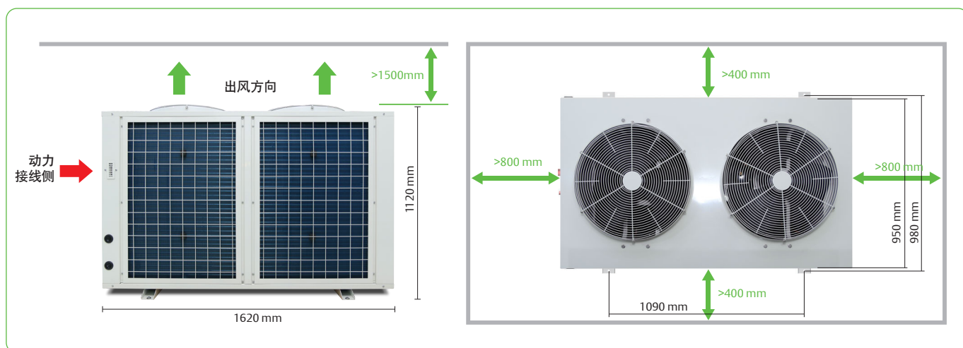
16HP机组安装间距
