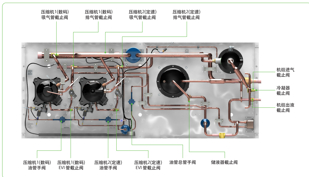
图12. 20HP机组的维修服务阀
