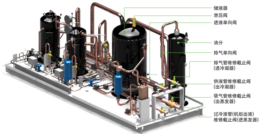
图10. 20HP机组的主要部件
