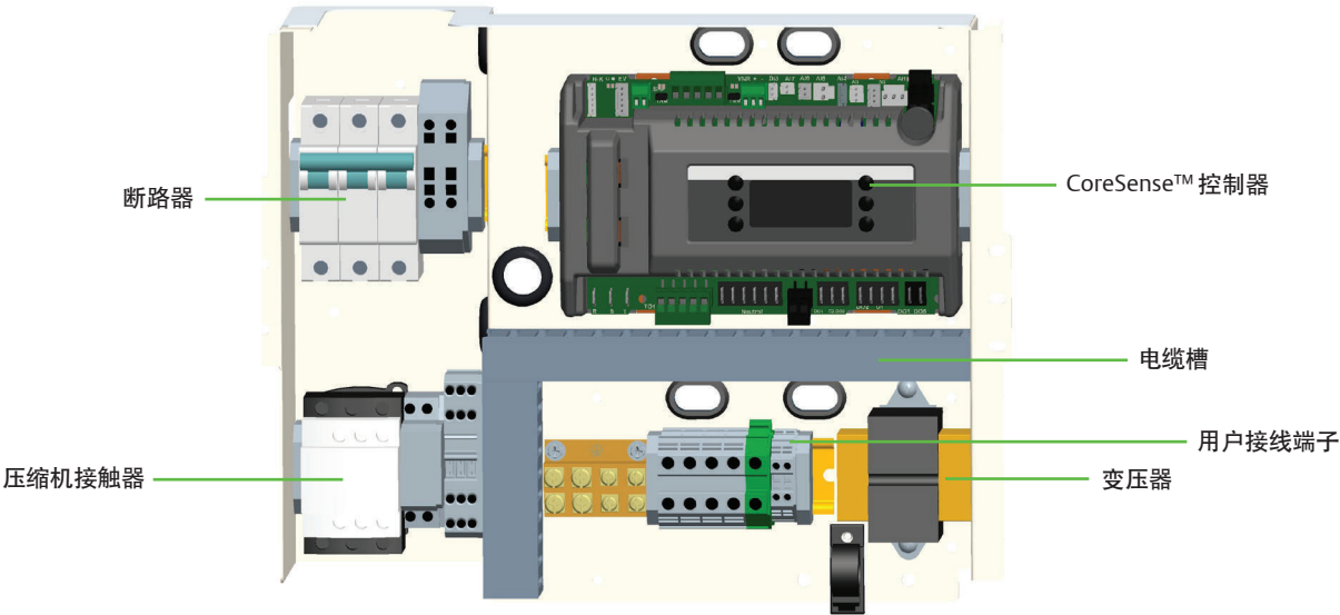
图4. CoreSense™和智能店模块外形
