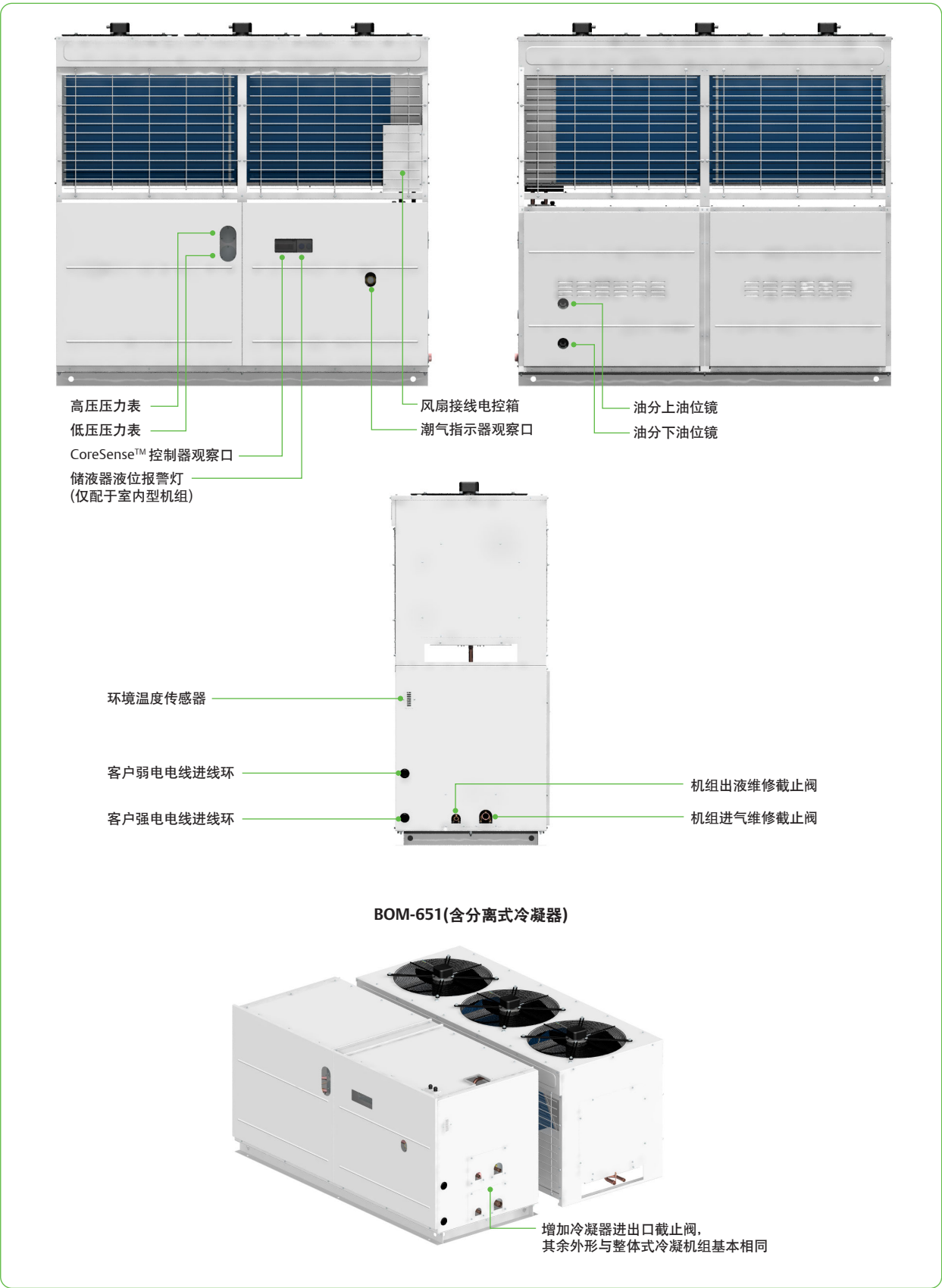
图9. 20HP机组外形
