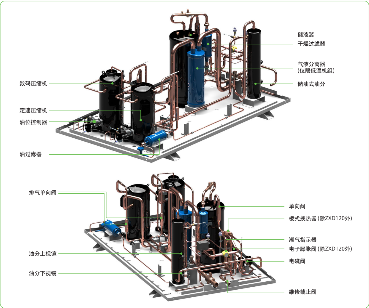
图6. 机组的主要部件
