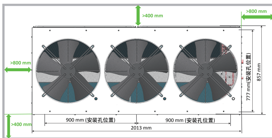
20HP机组安装间距
