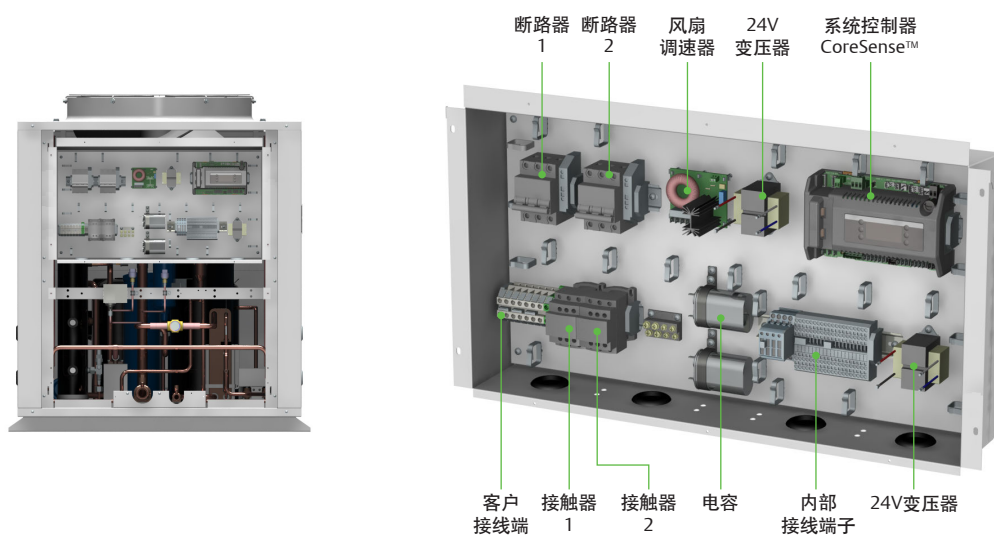
图7. 机组的电气模块
